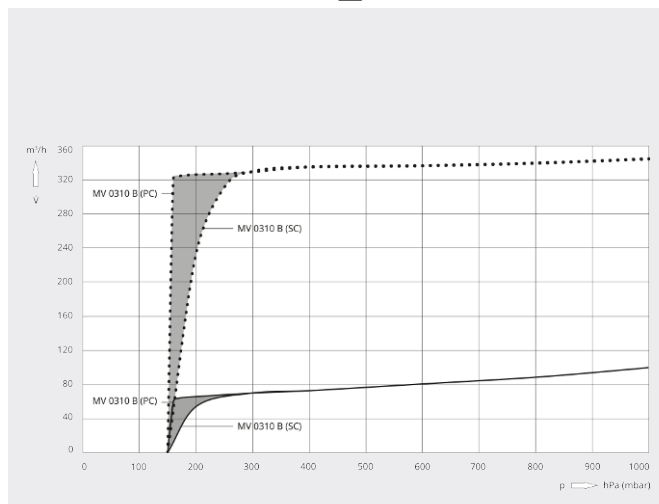
Pumpekapasitet
