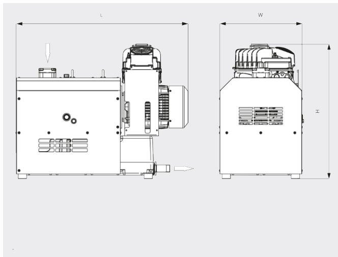
Dimensjonstegning
